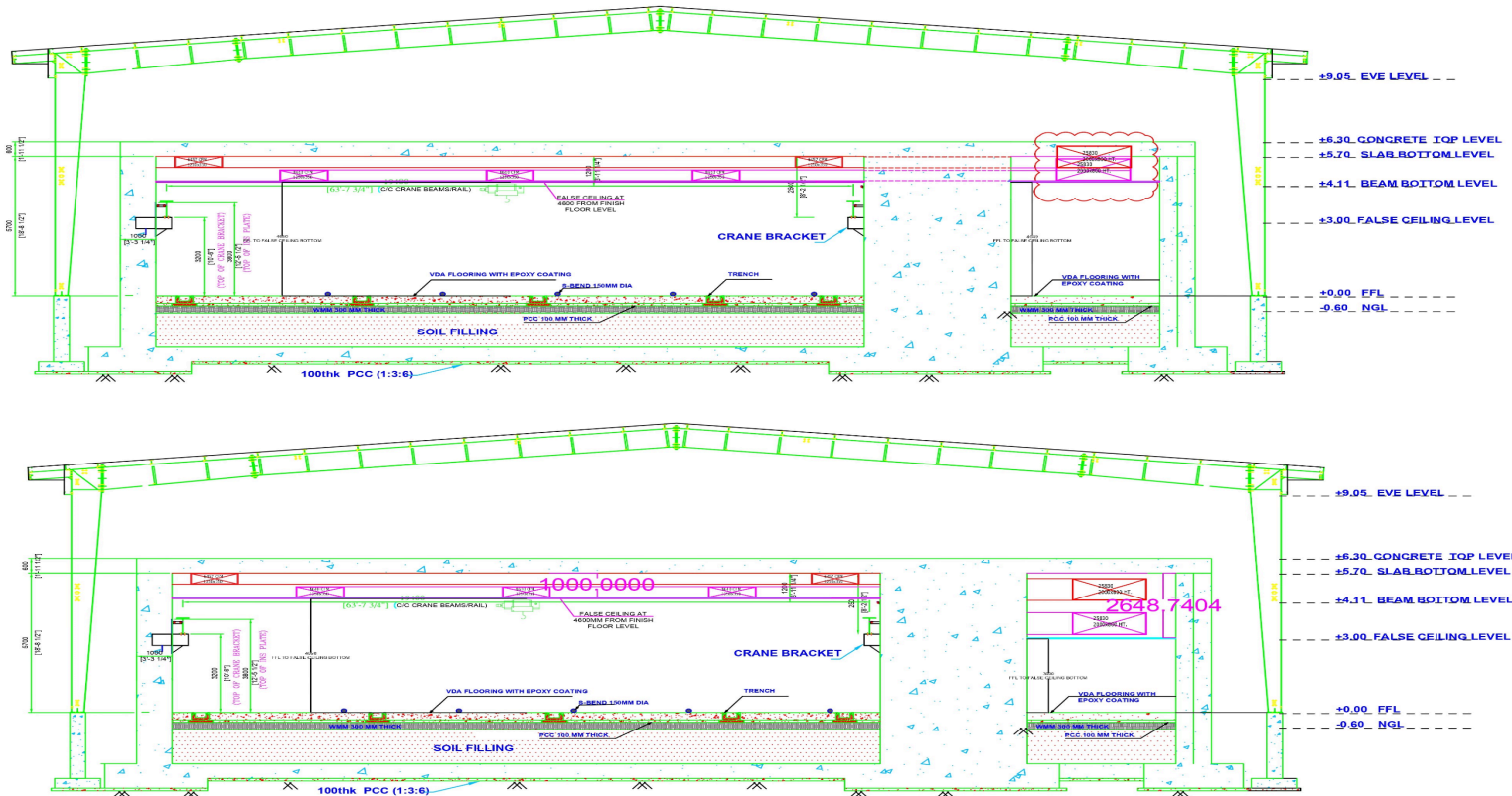
VIEW A-A
